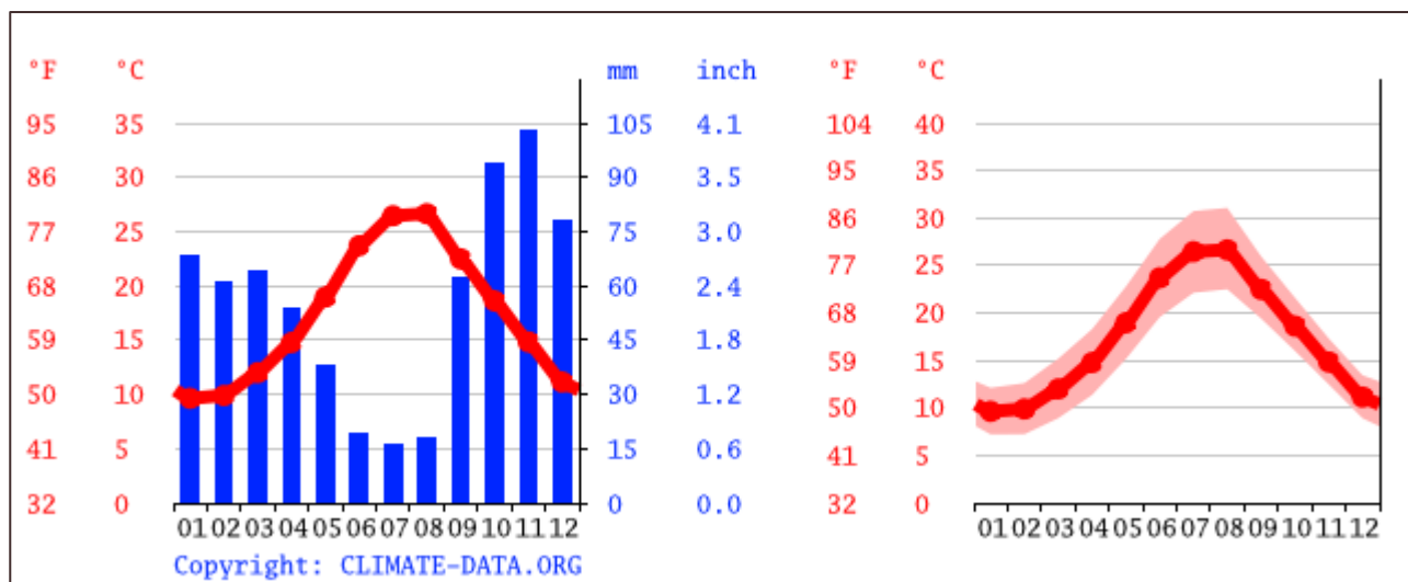
FIGURA 21: ANDAMENTO DELLE TEMPERATURE E DELLA PIOVOSITÀ
