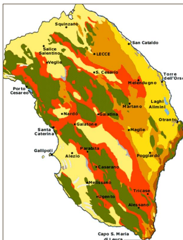
FIGURA 8: CONNESSIONE TRA IDROLOGIA E GEOMORFOLOGIA
