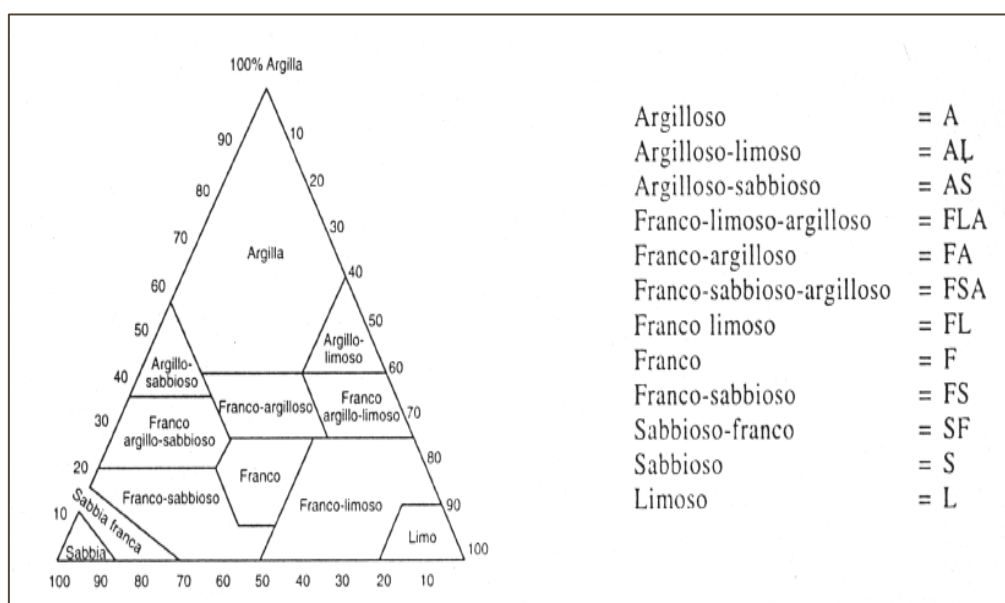
FIGURA 12: GLI INDICATORI DELLA QUALITÀ DEL SUOLO
