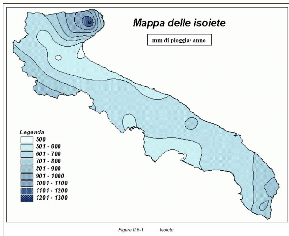
FIGURA 19: MAPPA DELLE ISOIETE
