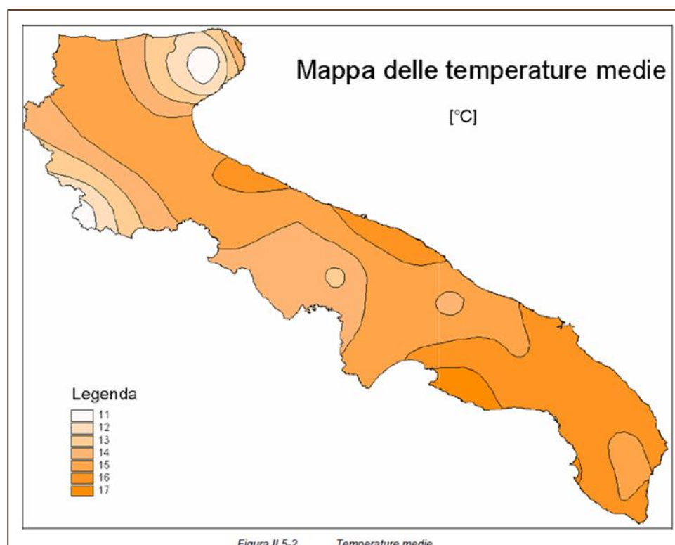
FIGURA 20: MAPPA DELLE TEMPERATURE MEDIE
