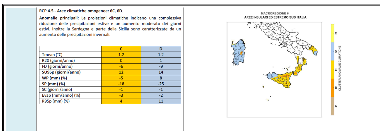
FIGURA 35: ANOMALIE SCENARIO RCP 4.5
