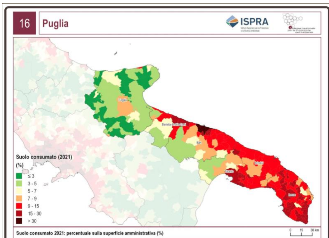
FIGURA 16: CONSUMO DI SUOLO AL 2021 – FONTE ISPRA
