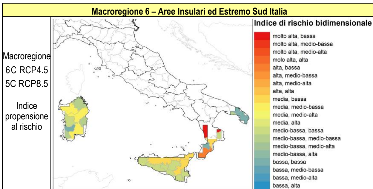
FIGURA 29: PROPENSIONE AL RISCHIO MACROREGIONE 6
