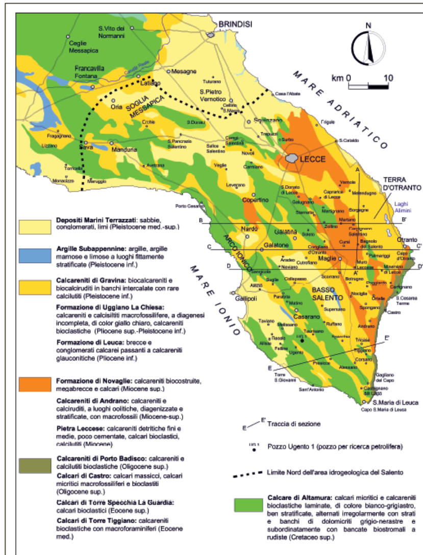
FIGURA 7: CARTA GEOLOGICA DELLA PROVINCIA DI LECCE
